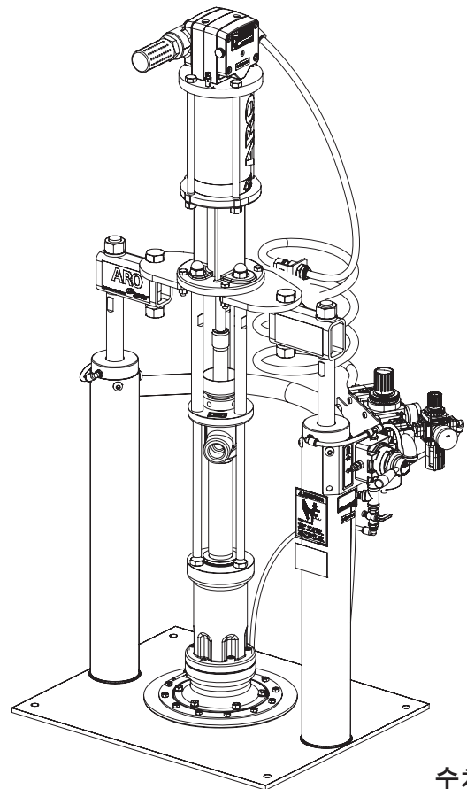
TP0423S2XXXXXXXXXX 램 패키지
